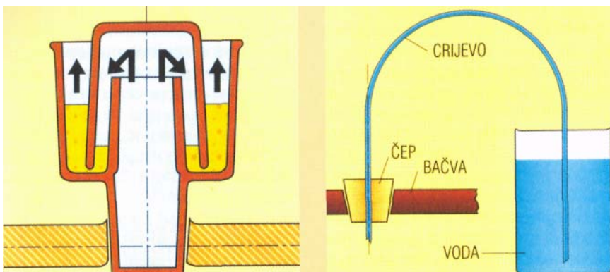
Shematski prikaz čepa s crijevom
