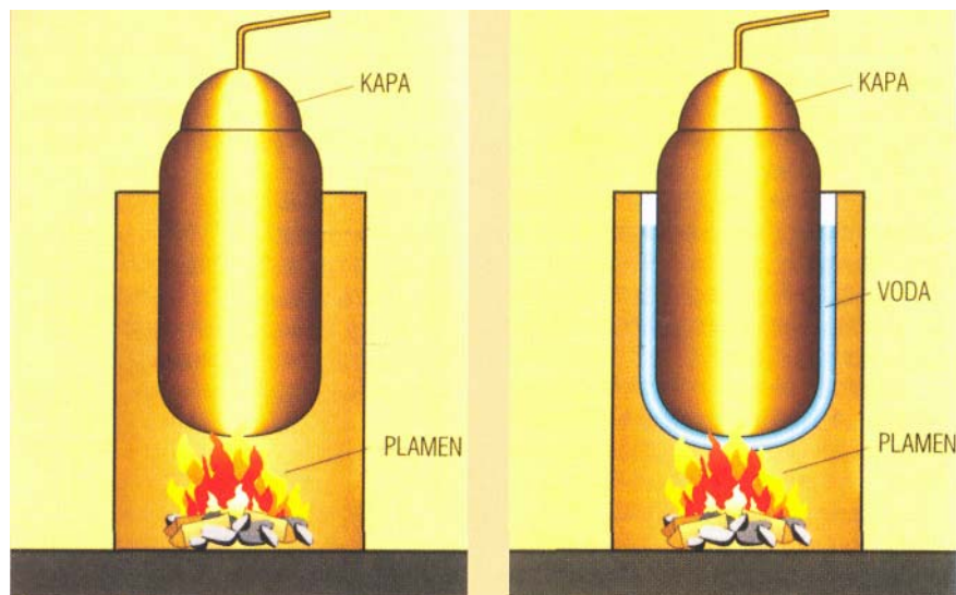
Slika 13: Shematski prikaz uređaja za pečenje s jednostrukom stijenkom
